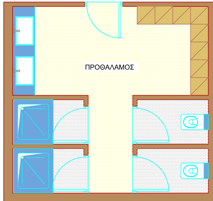
ΕΝΔΕΙΚΤΙΚΗ ΚΑΤΟΨΗ ΑΠΟΔΥΤΗΡΙΩΝ ΜΕ ΔΥΟ ΤΟΥΑΛΕΤΕΣ & ΔΥΟ ΝΤΟΥΣ
